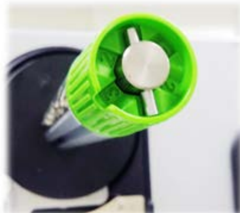
碳帶供應軸 張力 # 1
