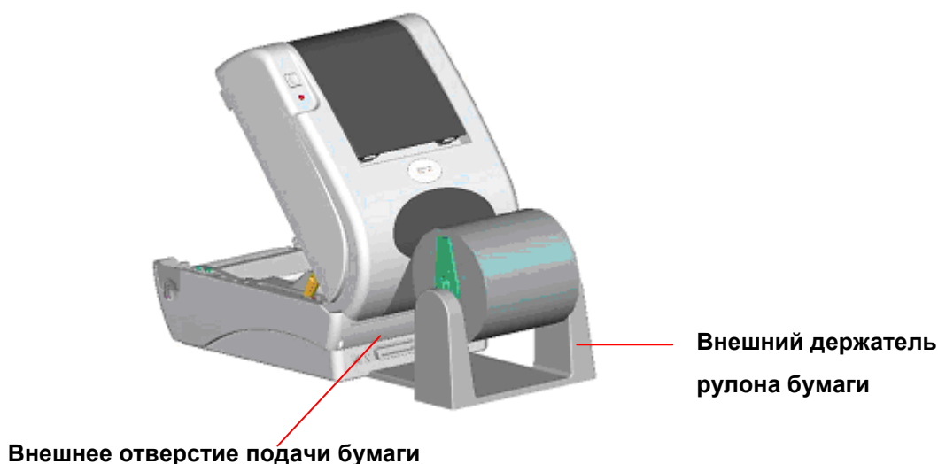
Рис. 10. Установка внешнего держателя рулона этикеток (I)
