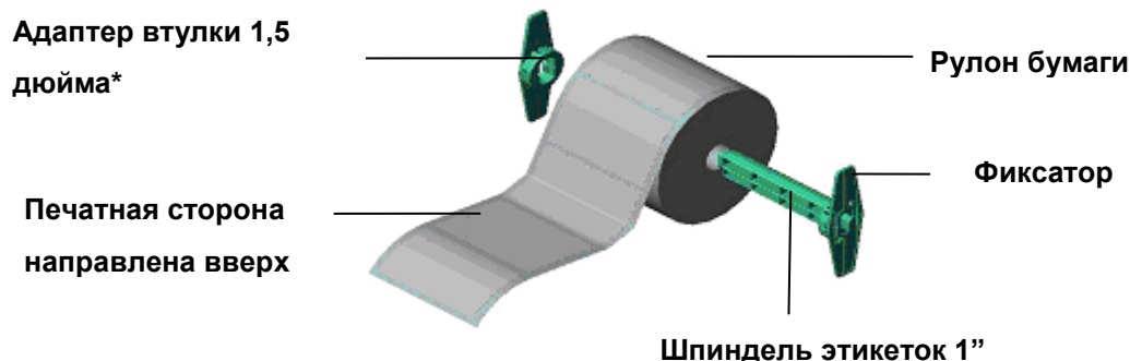
Рис. 6. Установка рулона этикеток (I)
