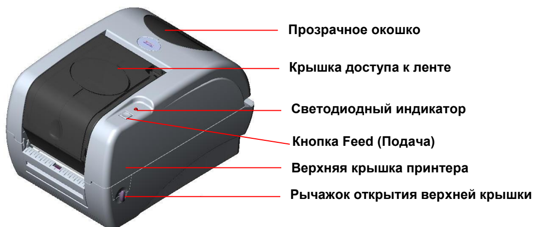
Рис. 1. Вид сверху и спереди
