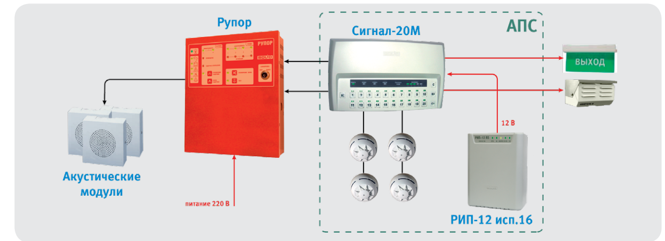
Рисунок 13. Пример СОУЭ 3-го типа с одной зоной оповещения
