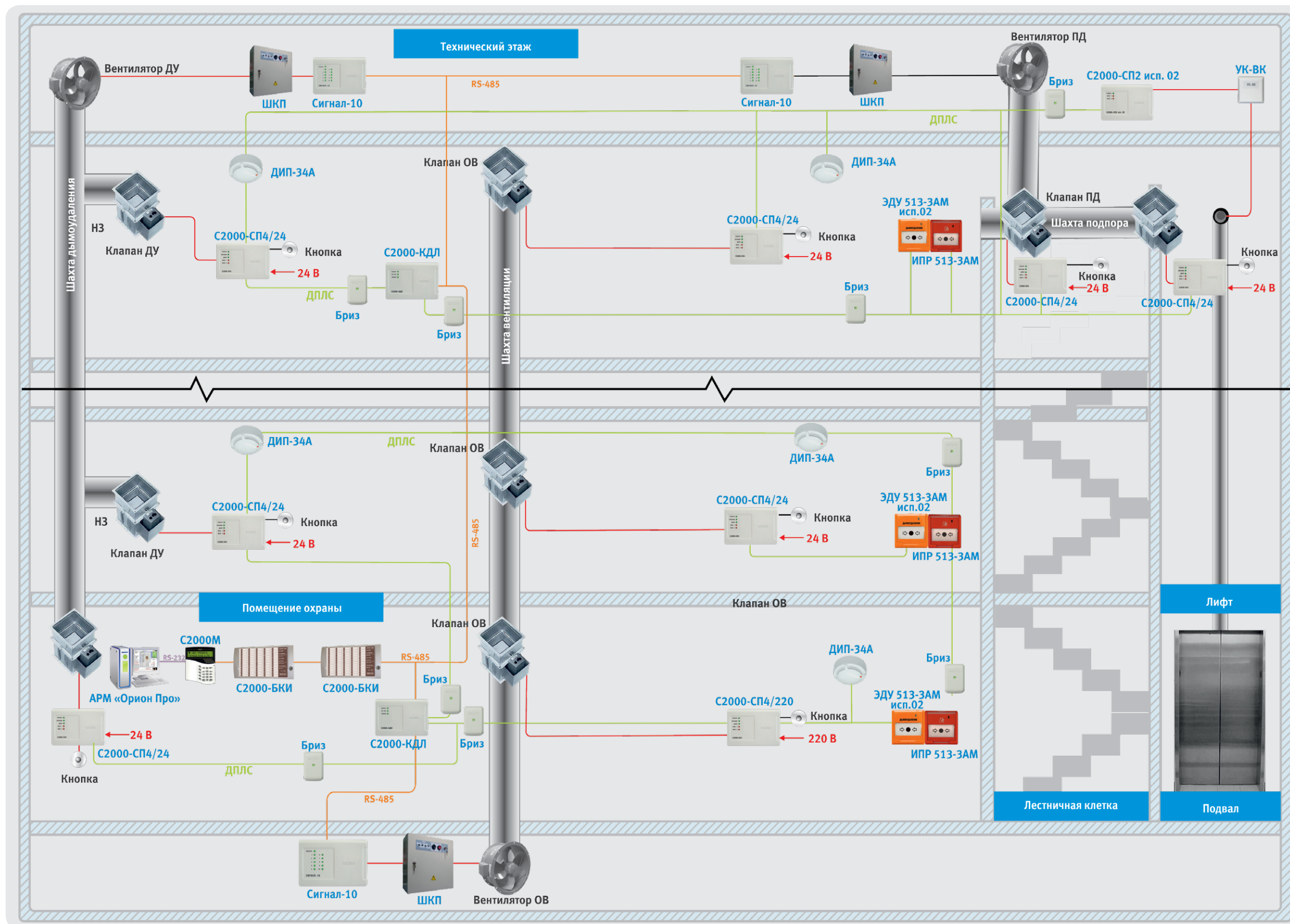
Рисунок 23. Структурная схема управления противопожарными клапанами
