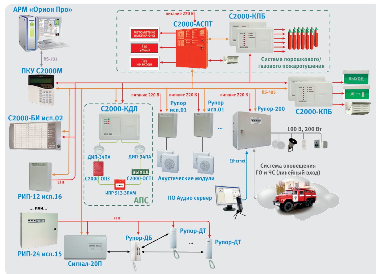
Рисунок 16. СОУЭ 5-го типа с комплексом обратной связи, входящим в состав
