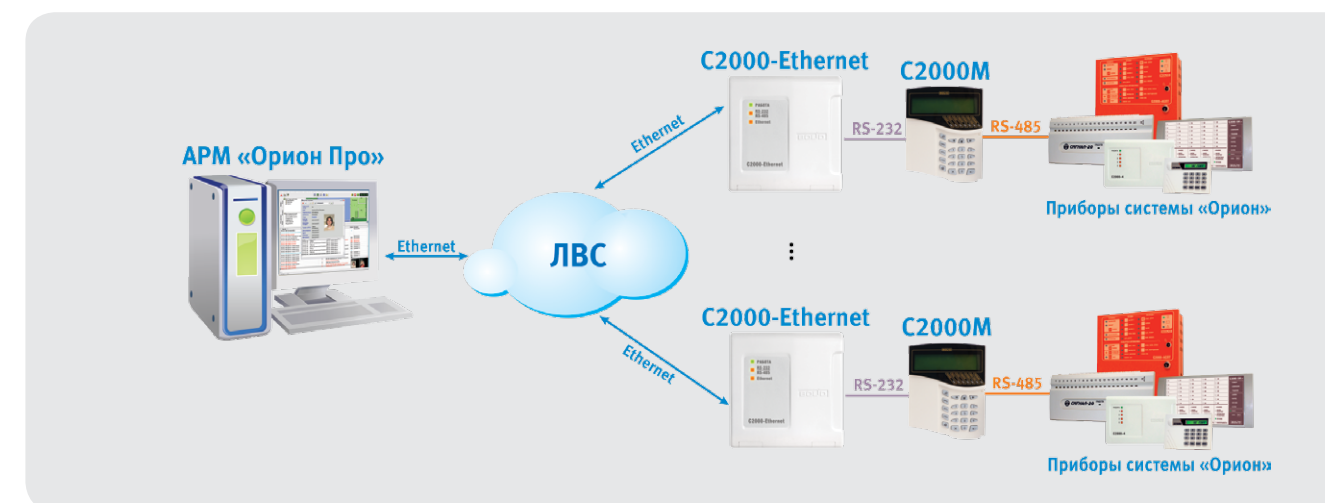
Рисунок 71. Типовая схема работы «С2000-Ethernet» по протоколу «Орион Про»
