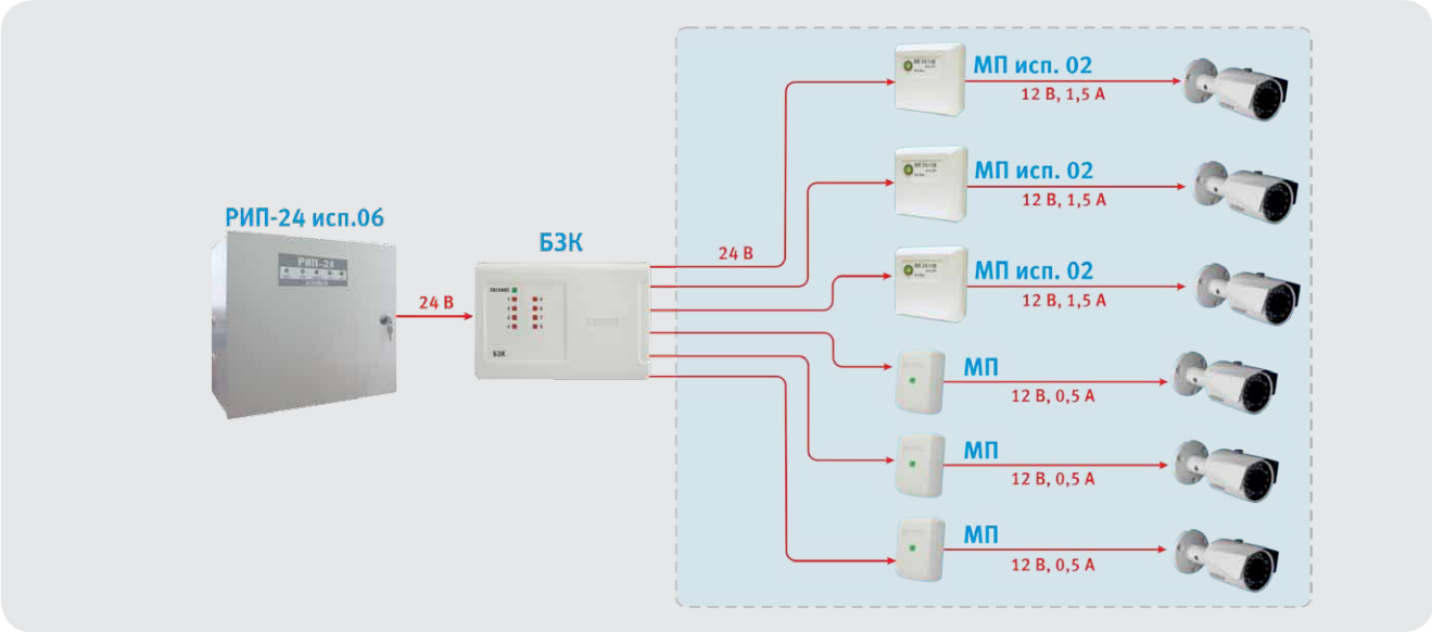
Рисунок 58. Организация электропитания системы видеонаблюдения
