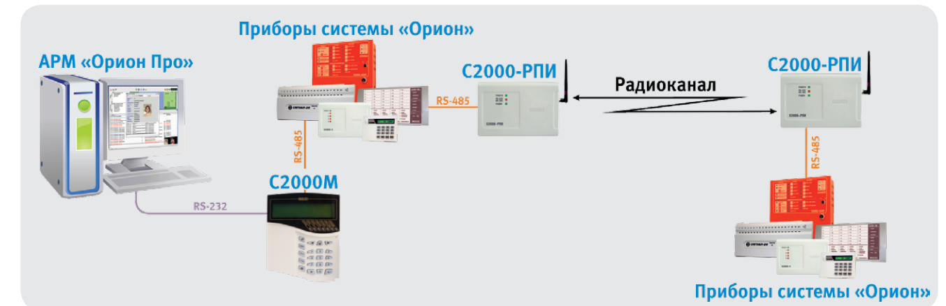
Рисунок 83. Структурная схема использования «С2000-РПИ» с АРМ «Орион Про» и «С2000М», соединение «точка-точка»
