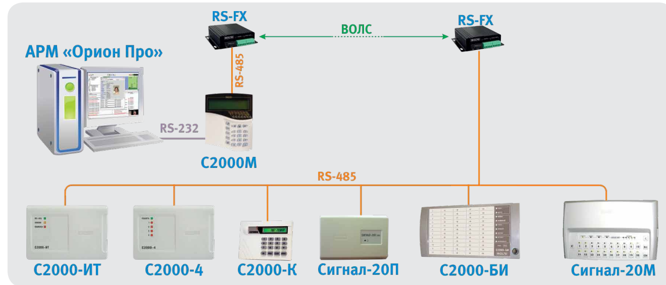
Рисунок 82. Структурная схема использования преобразователей RS-FX с АРМ «Орион Про» и «С2000М»
