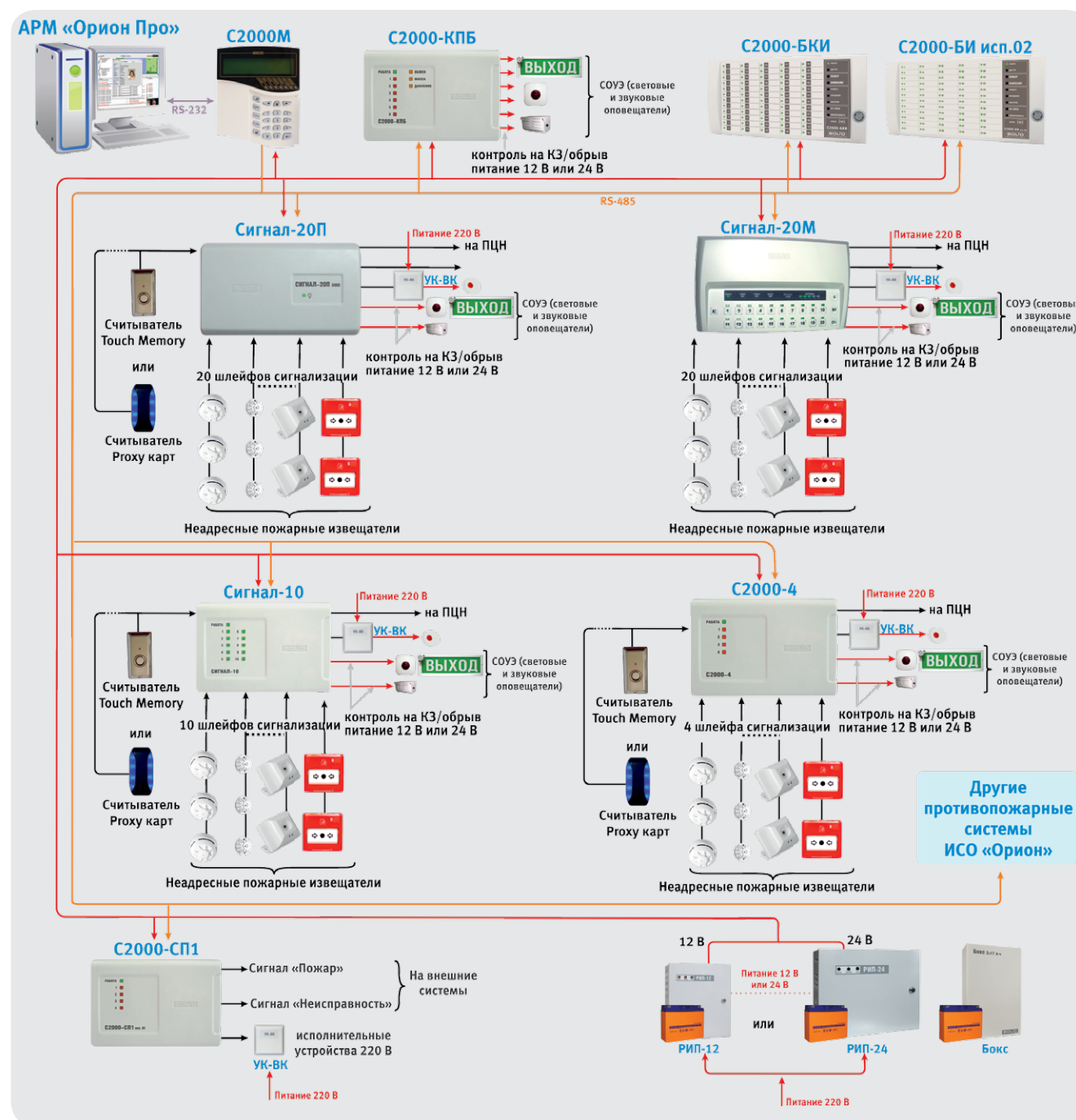
Рисунок 4. Неадресная система пожарной сигнализации в ИСО «Орион»
