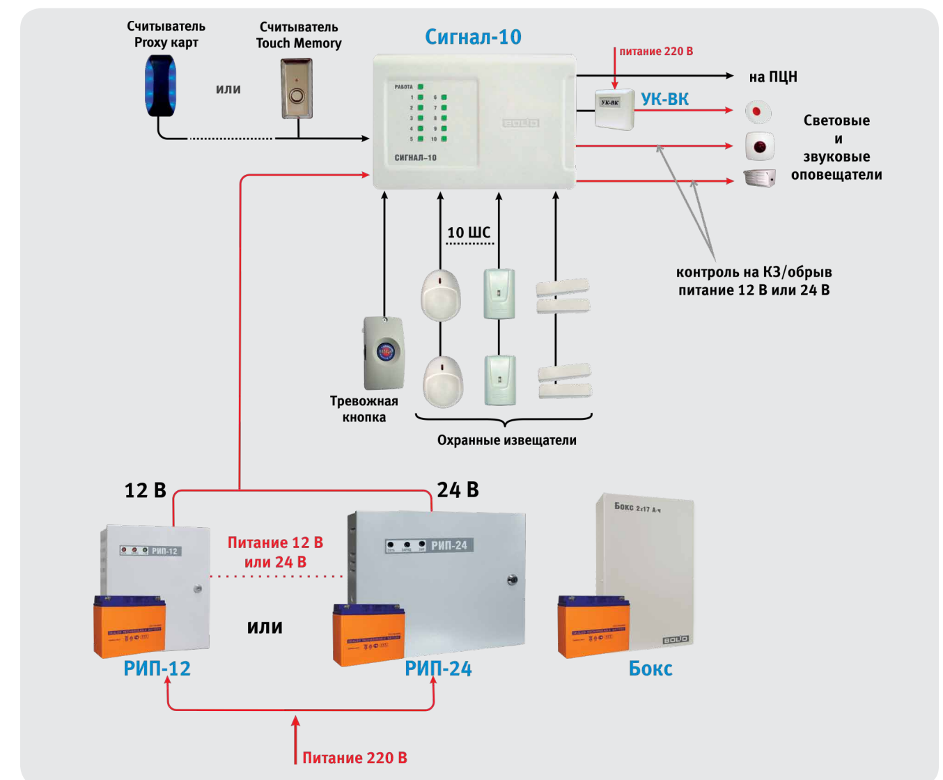
Рисунок 26. Автономное использование прибора «Сигнал-10»
