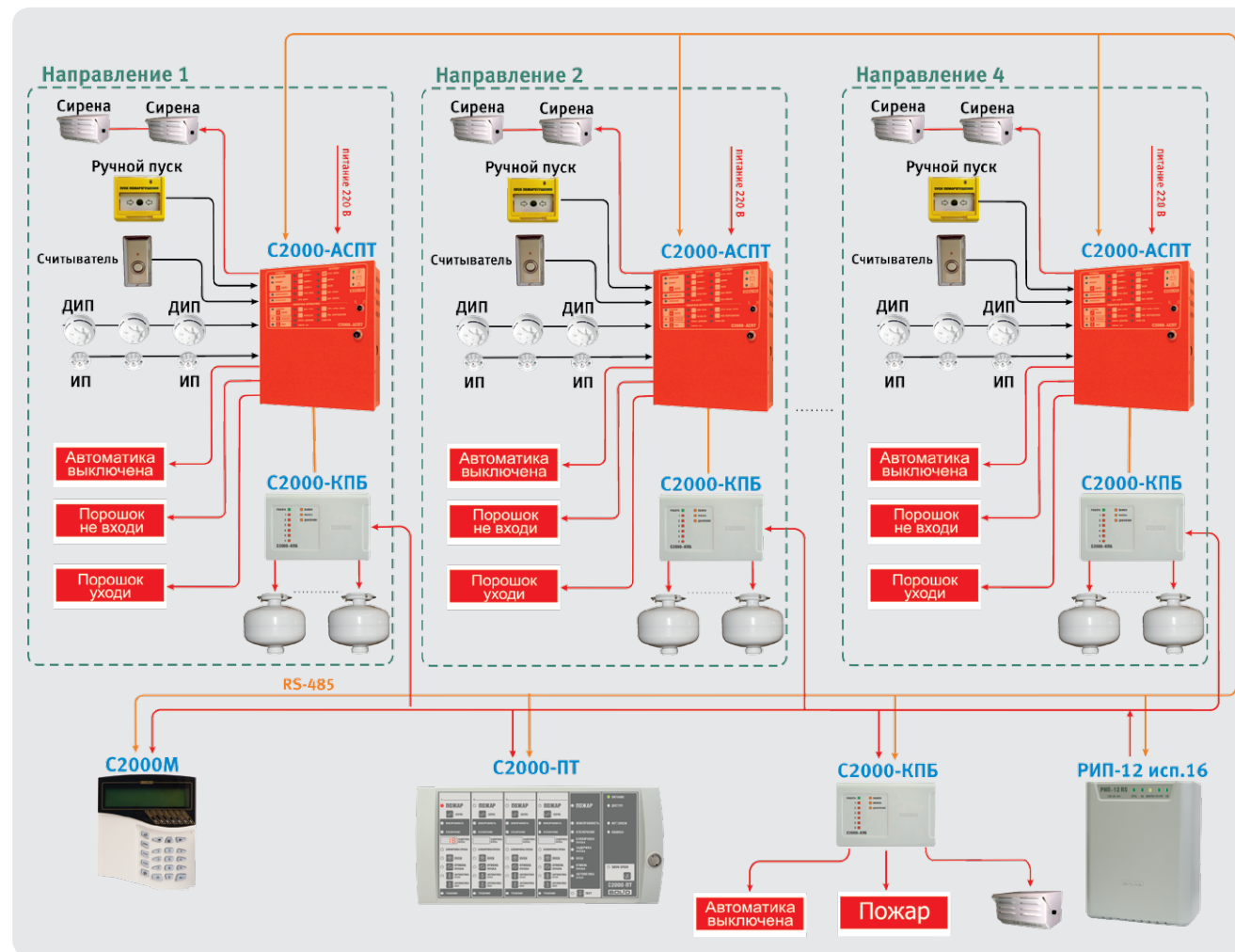
Рисунок 19. Система порошкового пожаротушения
