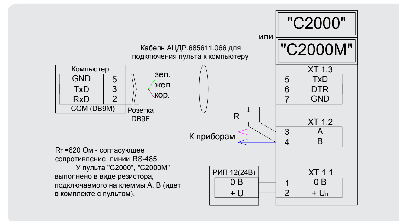
Рисунок 67. Схема подключения пульта «С2000»/ «С2000М» к персональному компьютеру с АРМ «Орион Про»
