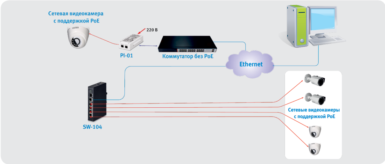
Рисунок 59. Организация электропитания сетевой системы видеонаблюдения с использованием технологии PoE
