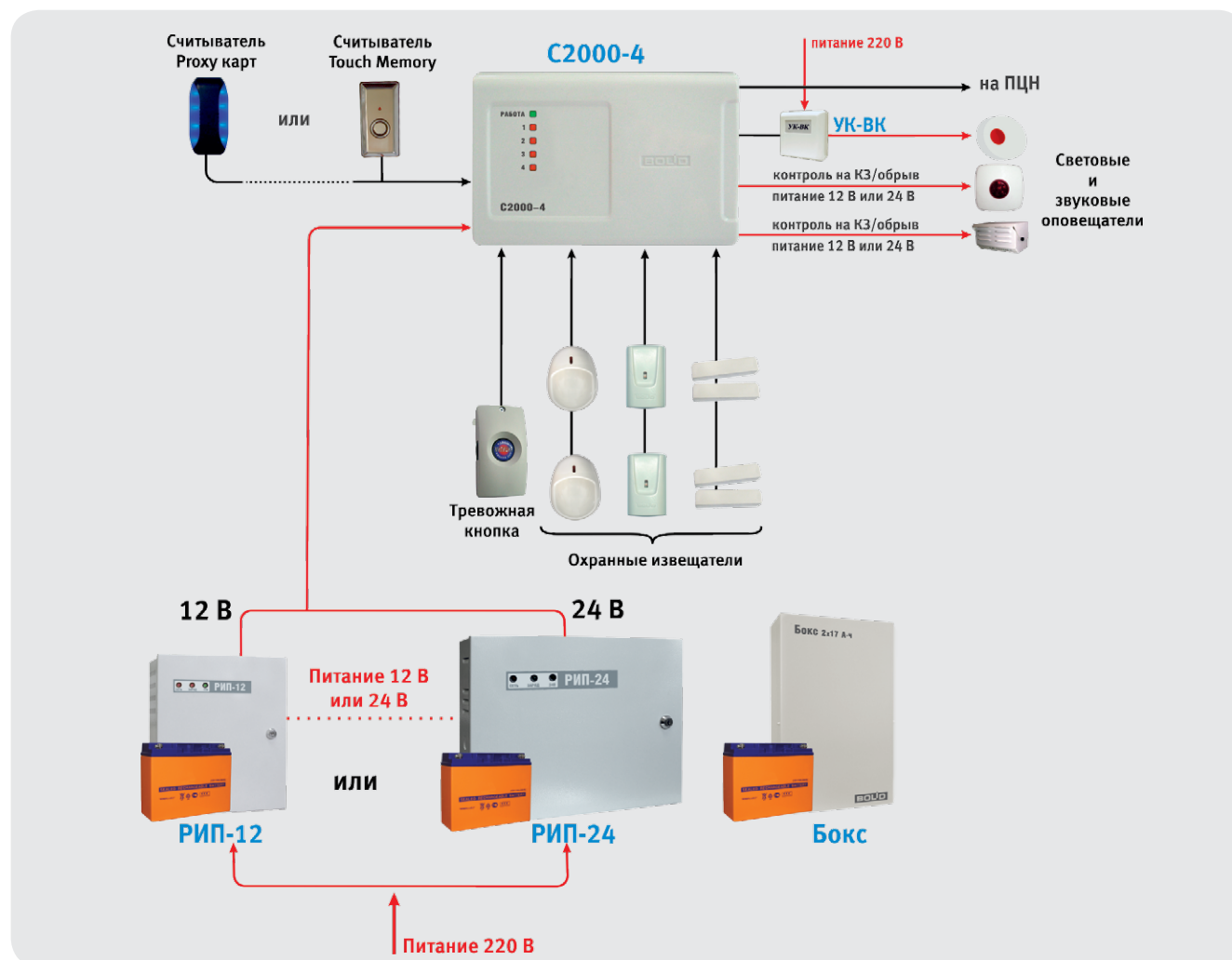
Рисунок 25. Автономное использование прибора «С2000-4»
