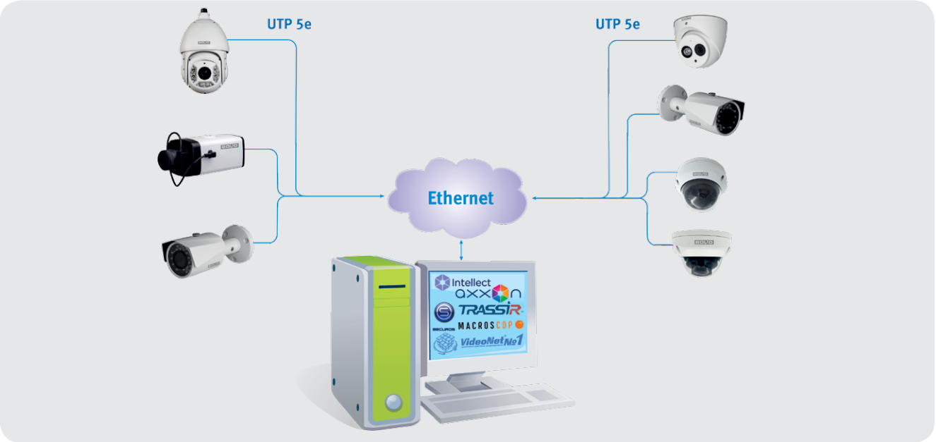
Рисунок 53. Сетевое видеонаблюдение напрямую с сетевых камер с удаленным рабочим местом на сторонних системах видеорегистрации
