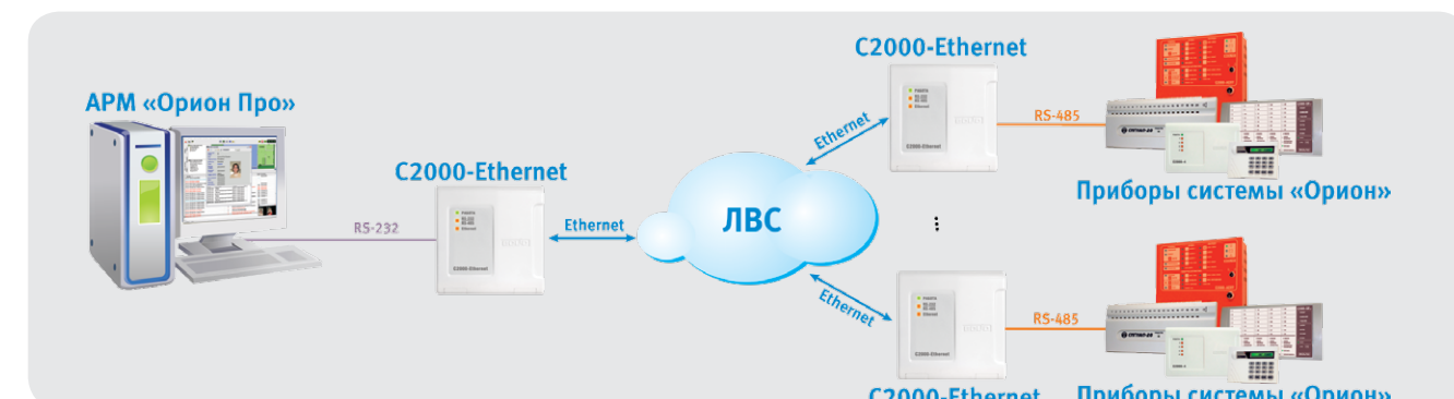
Рисунок 88. Типовая схема работы «C2000-Ethernet» по протоколу «Орион»
