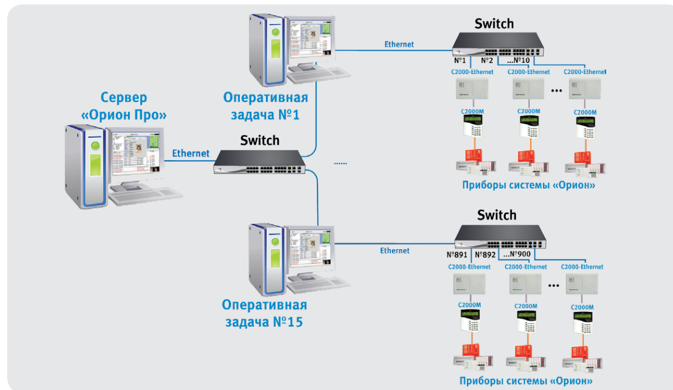
Рисунок 73. Пример построения системы с использованием «C2000-Ethernet» на 900 объектах
