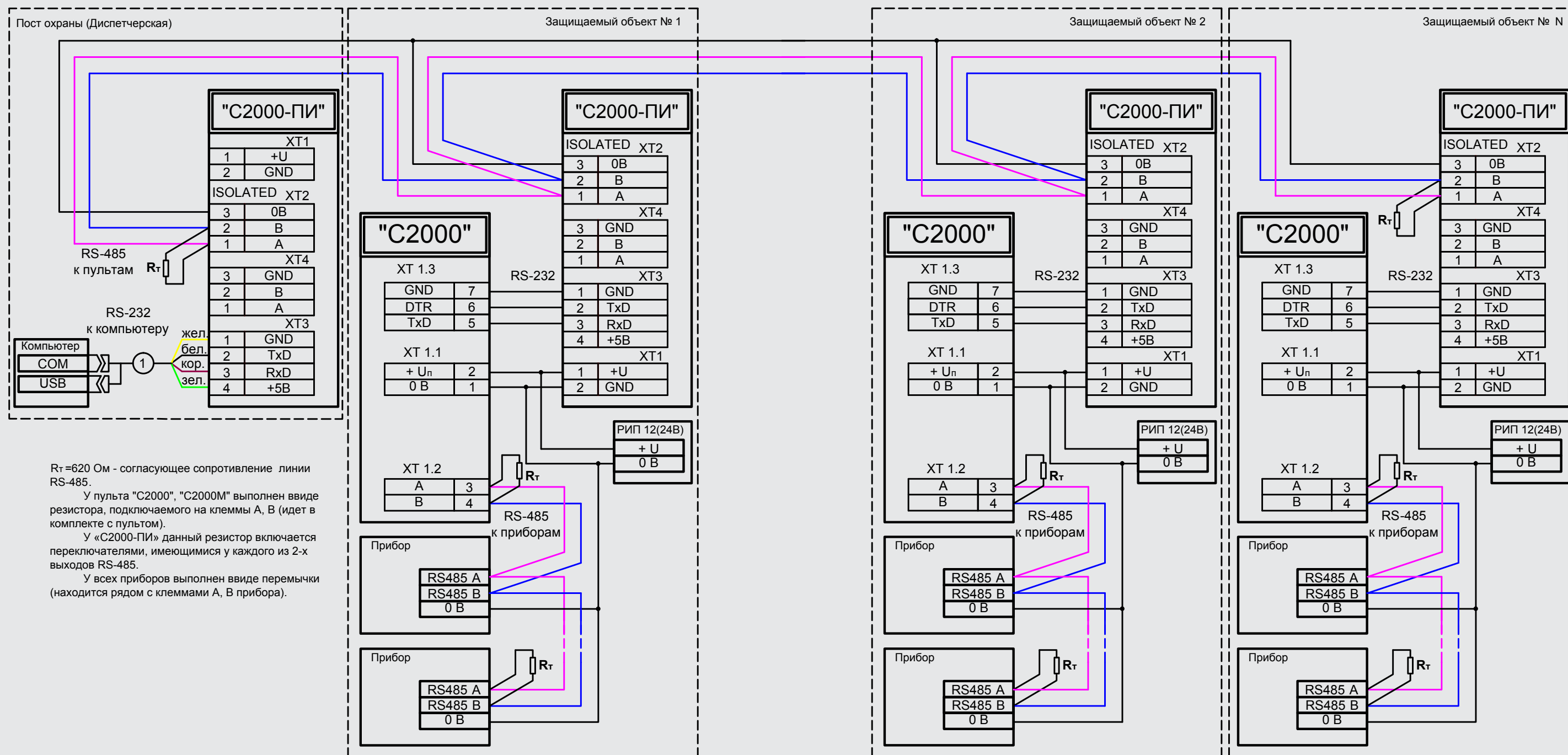
Рисунок 69. Схема подключения нескольких пультов к
