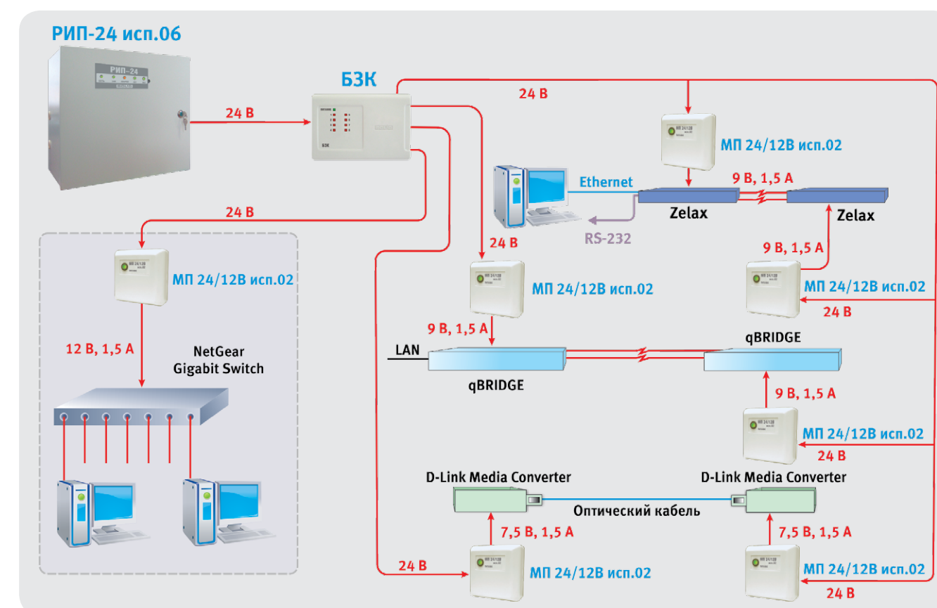
Рисунок 47. Электропитание сетевого каналаобразующего оборудования
