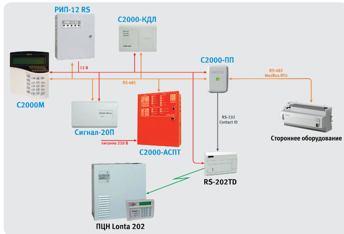
Рисунок 63. Применение «С2000-ПП» в ведомом режиме
