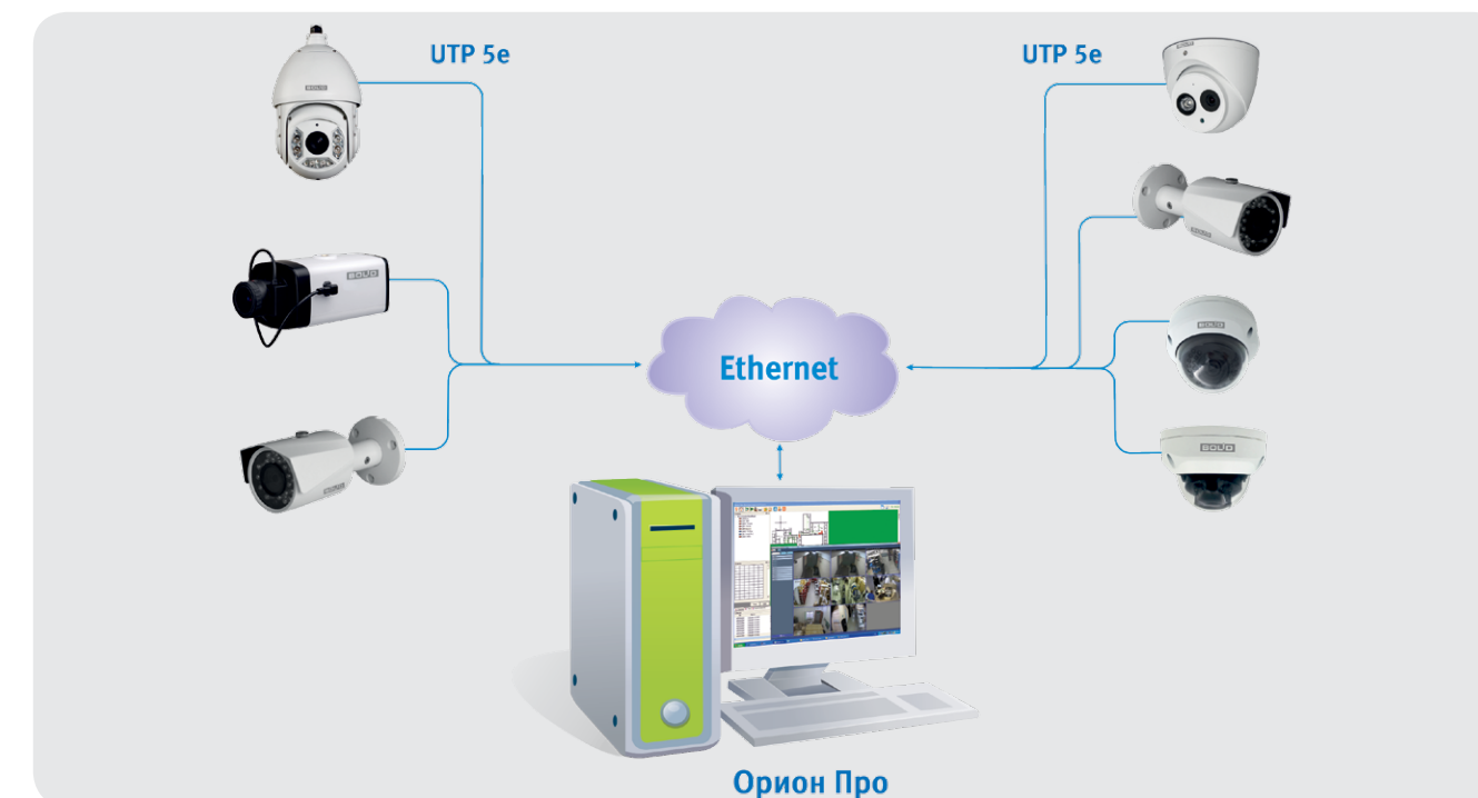
Рисунок 52. Сетевое видеонаблюдение напрямую с сетевых камер с удаленным рабочим местом на АРМ Орион Про
