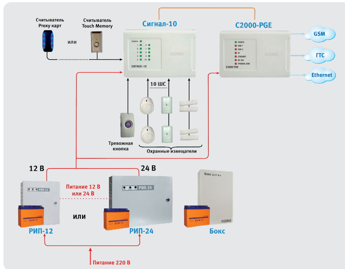
Рисунок 29. Система охранной сигнализации на базе прибора «Сигнал-10» и устройства «C2000-PGE»
