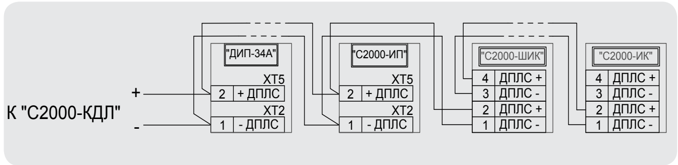
Рисунок 90. Схема подключения адресных извещателей в ДПЛС с топологией построения «шина»
