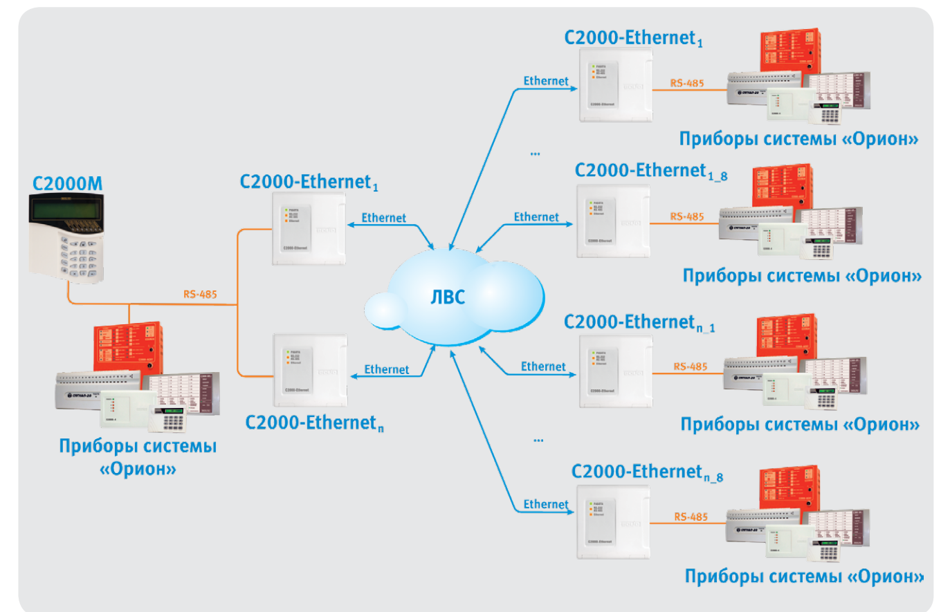
Рисунок 81. Структурная схема использования «С2000-Ethernet» с «С2000М»
