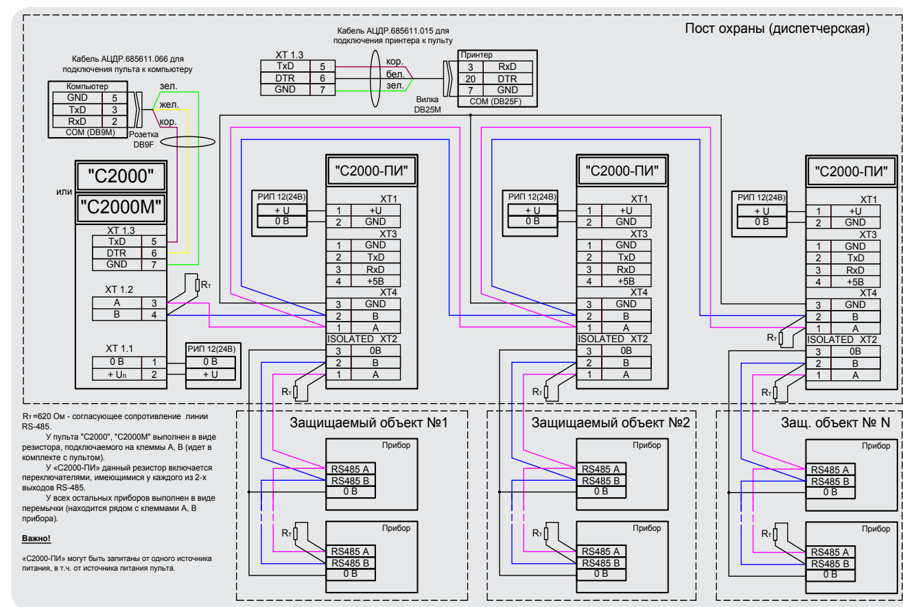
Рисунок 80. Построение сети RS-485 с топологией «звезда» при помощи повторителей
