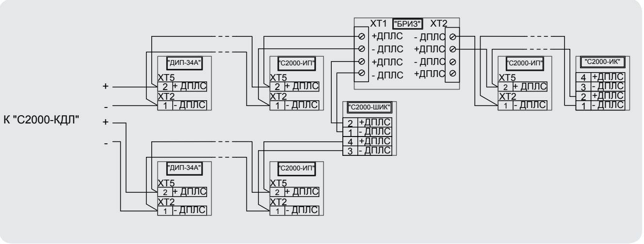
Рисунок 92. Схема подключения адресных извещателей в ДПЛС с топологией построения «кольцо»
