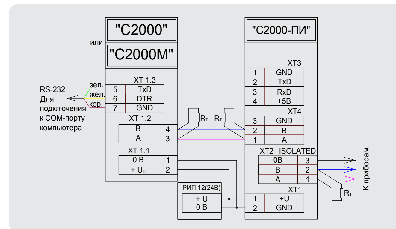
Рисунок 68. Схема подключения пультов «С2000»/ «С2000М» к персональному компьютеру с АРМ «Орион Про» с гальванической изоляцией интерфейса RS-485
