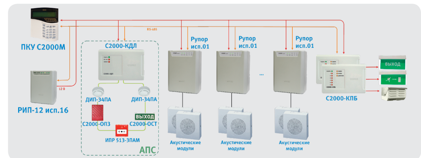
Рисунок 14. Пример СОУЭ 3-го типа с несколькими зонами оповещения
