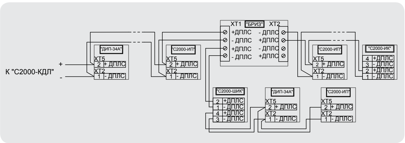
Рисунок 91. Схема подключения адресных устройств в ДПЛС с топологией построения «дерево»
