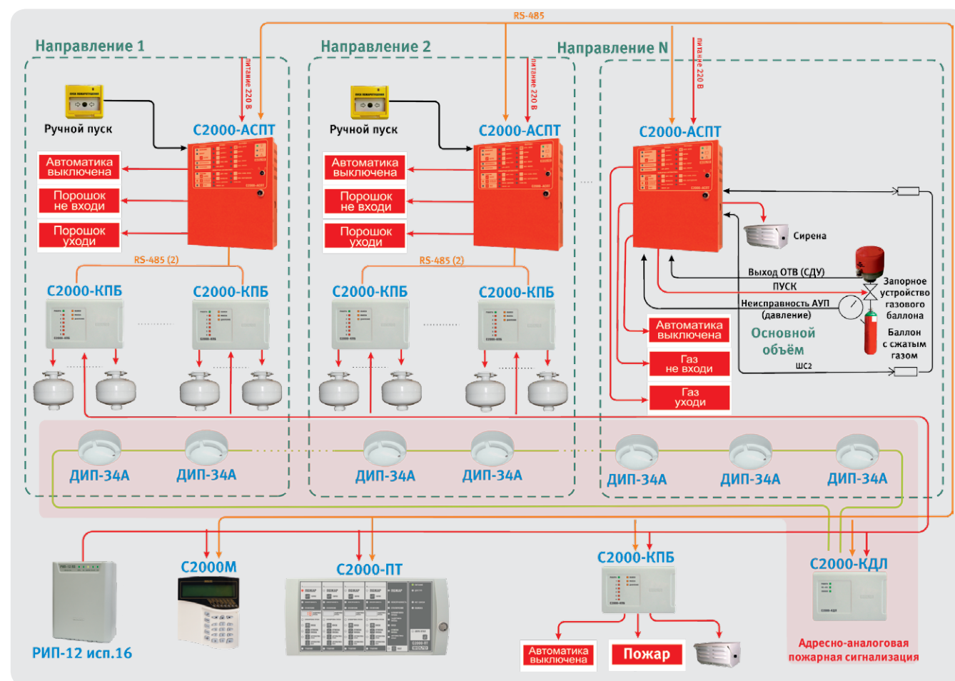
Рисунок 21. Система газового и порошкового тушения с использованием адресно-аналоговой пожарной сигнализации
