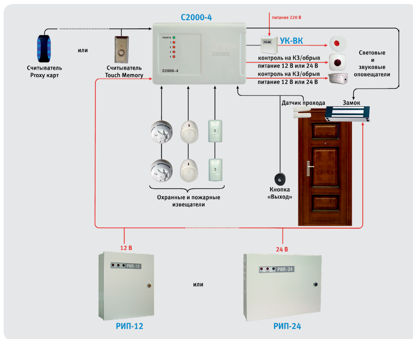
Рисунок 42. «С2000-4» с функционалом контроля доступа
