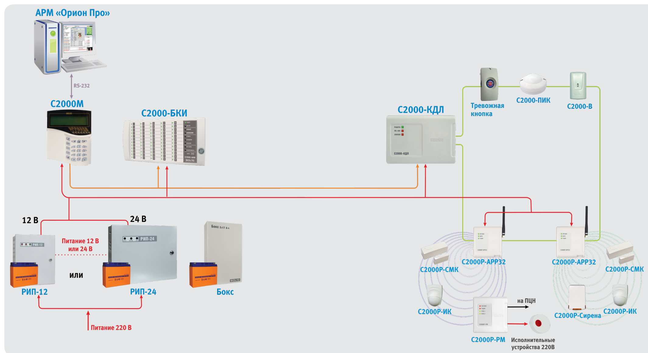
Рисунок 32. Адресная радиоканальная система на основе «С2000Р-АРР32»
