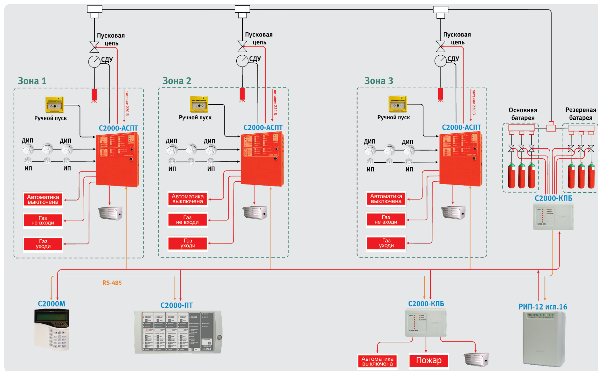
Рисунок 18. Централизованная система автоматического пожаротушения с газовой батареей
