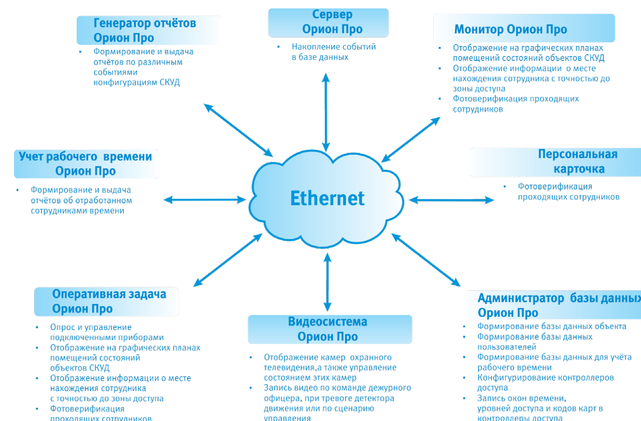
Рисунок 46. Функционал модулей программного обеспечения
