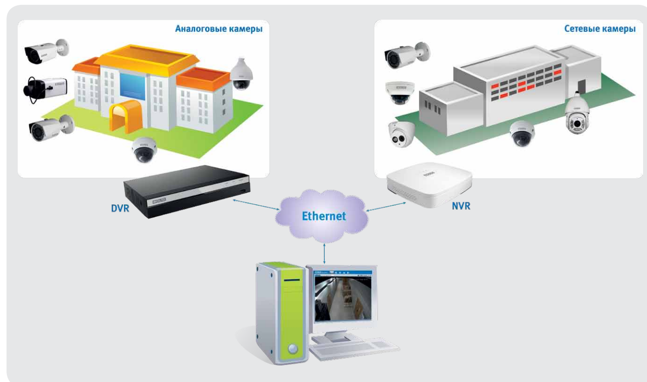
Рисунок 50. Аналоговое и/или сетевое видеонаблюдение с удаленным рабочим местом через программу Web-Browser
