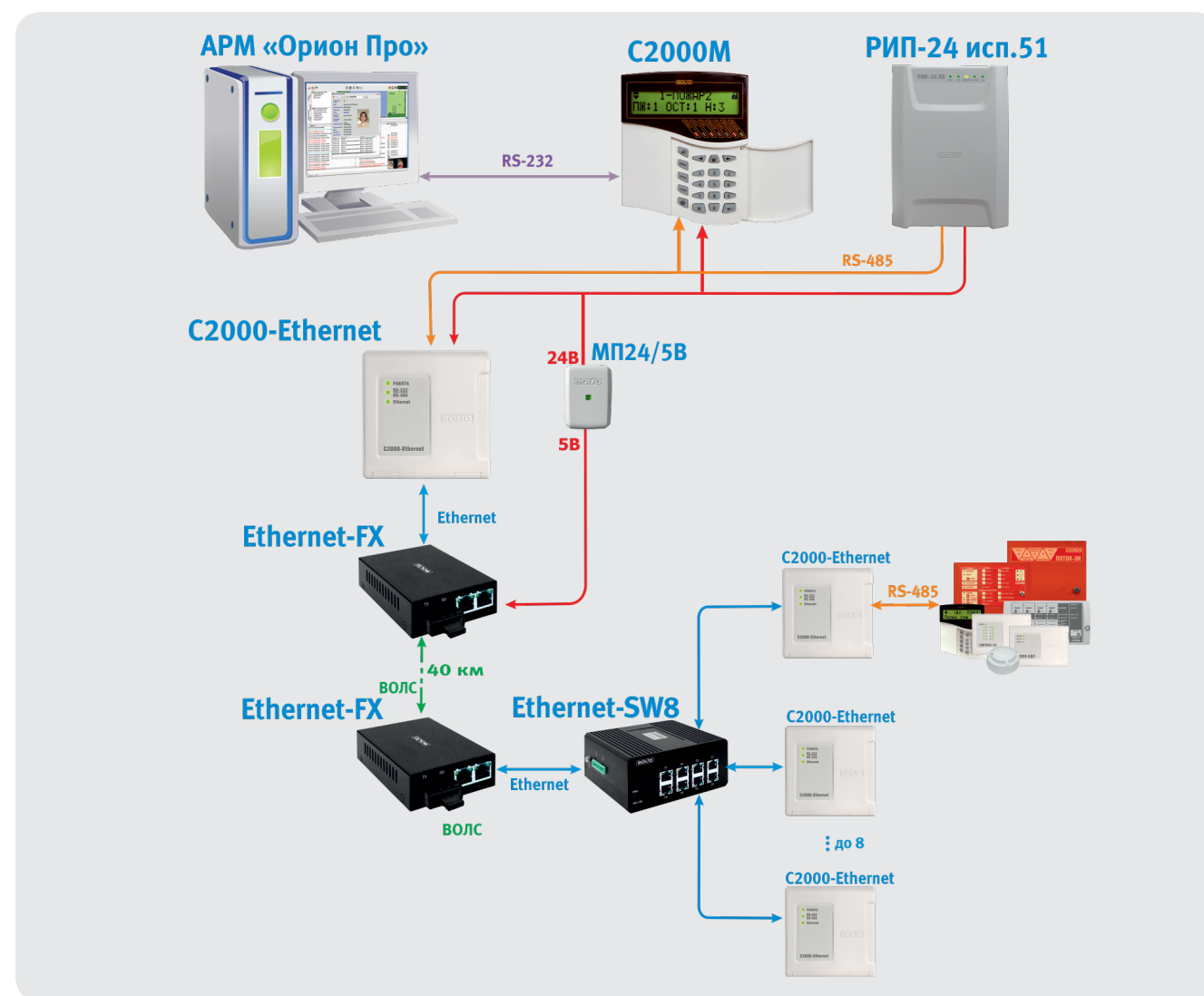
Рисунок 93. Каналообразующее оборудование для систем пожарной сигнализации и автоматики
