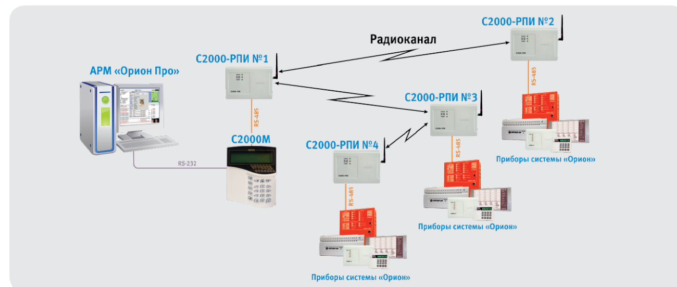
Рисунок 85. Структурная схема использования «C2000-RPI» с АРМ «Орион» и «C2000М», соединение «точка-многоточие» с ретрансляцией
