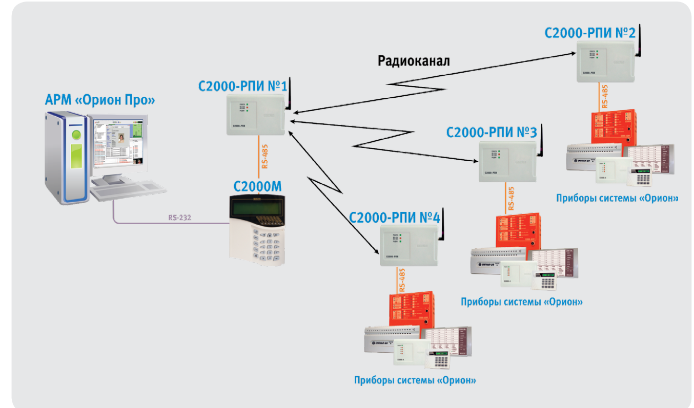
Рисунок 84. Структурная схема использования «С2000-РПИ» с АРМ «Орион Про» и «С2000М», соединение «точка-многоточие»
