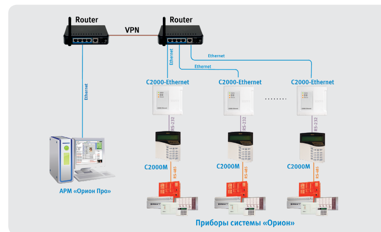
Рисунок 72. Пример использования «С2000-Ethernet» в глобальных сетях
