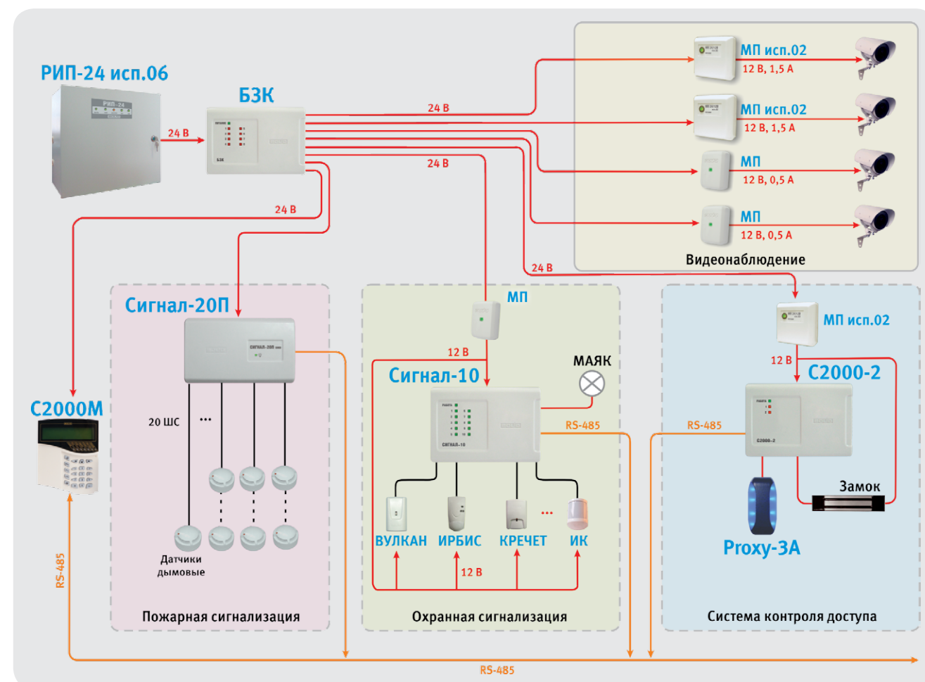
Рисунок 61. Организация электропитания интегрированных систем
