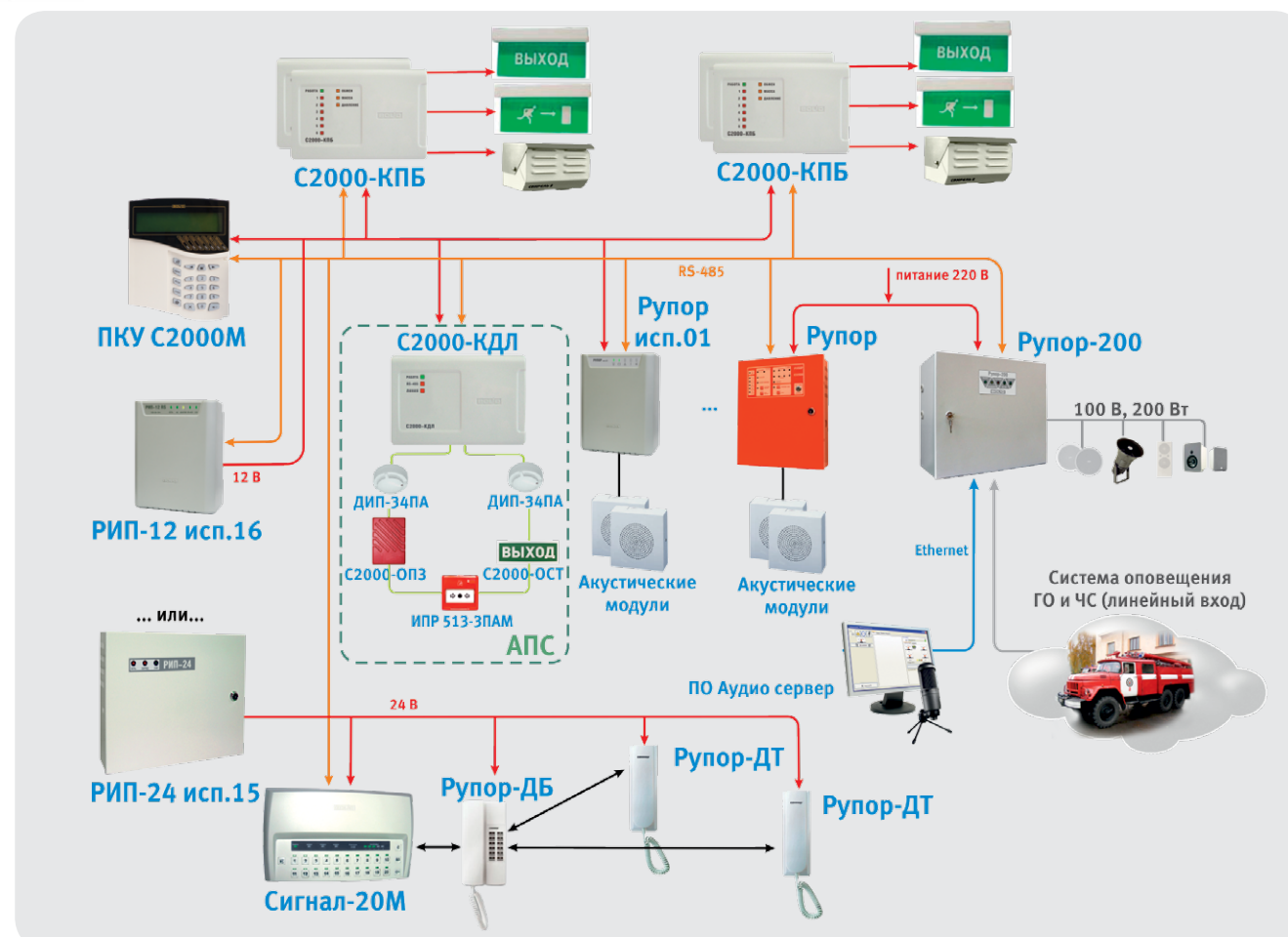
Рисунок 15. Пример СОУЭ 4-го типа с автономным комплексом обратной связи ИСО «Орион»
