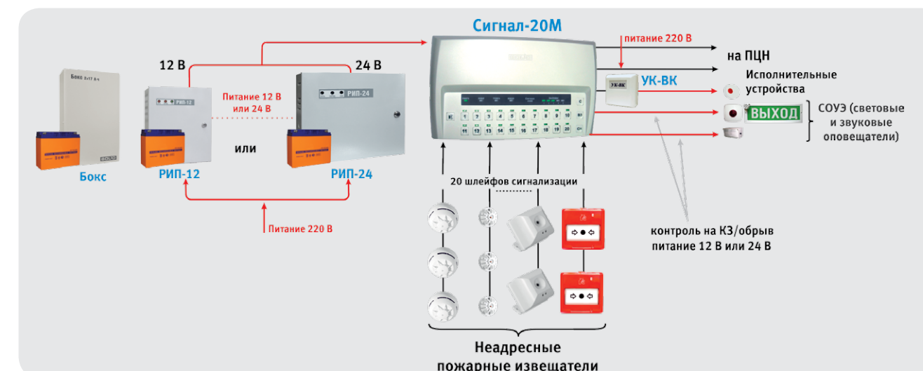
Рисунок 3. Использование прибора «Сигнал-20М» в автономном режиме
