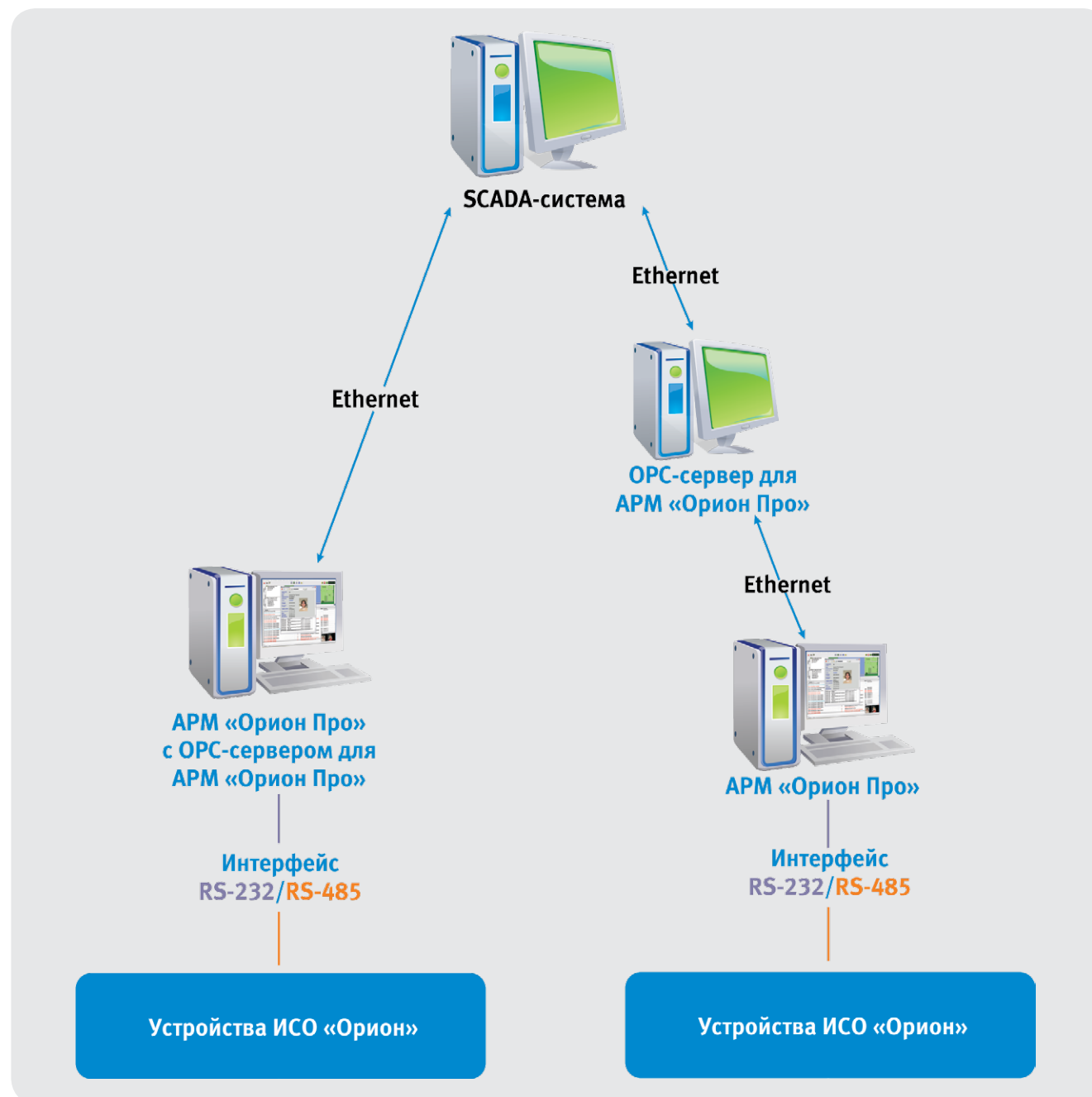
Рисунок 66. Передача данных в SCADA-системе
