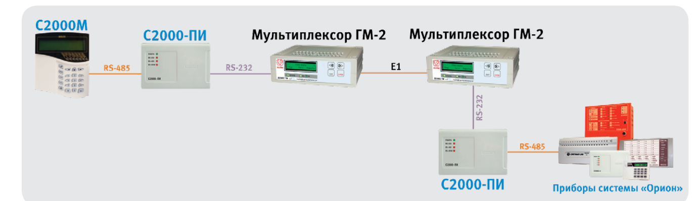
Рисунок 77. Структурная схема использования мультиплексора «ГМ-2» с пультом «C2000M»
