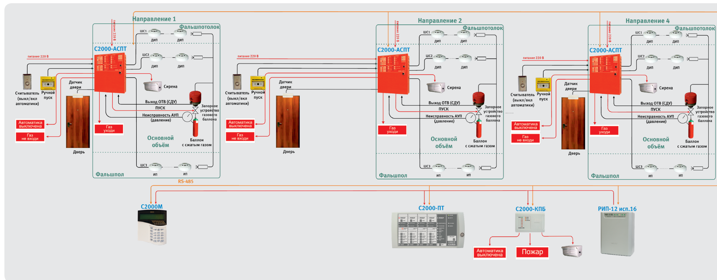
Рисунок 17. Распределенная установка газового пожаротушения
