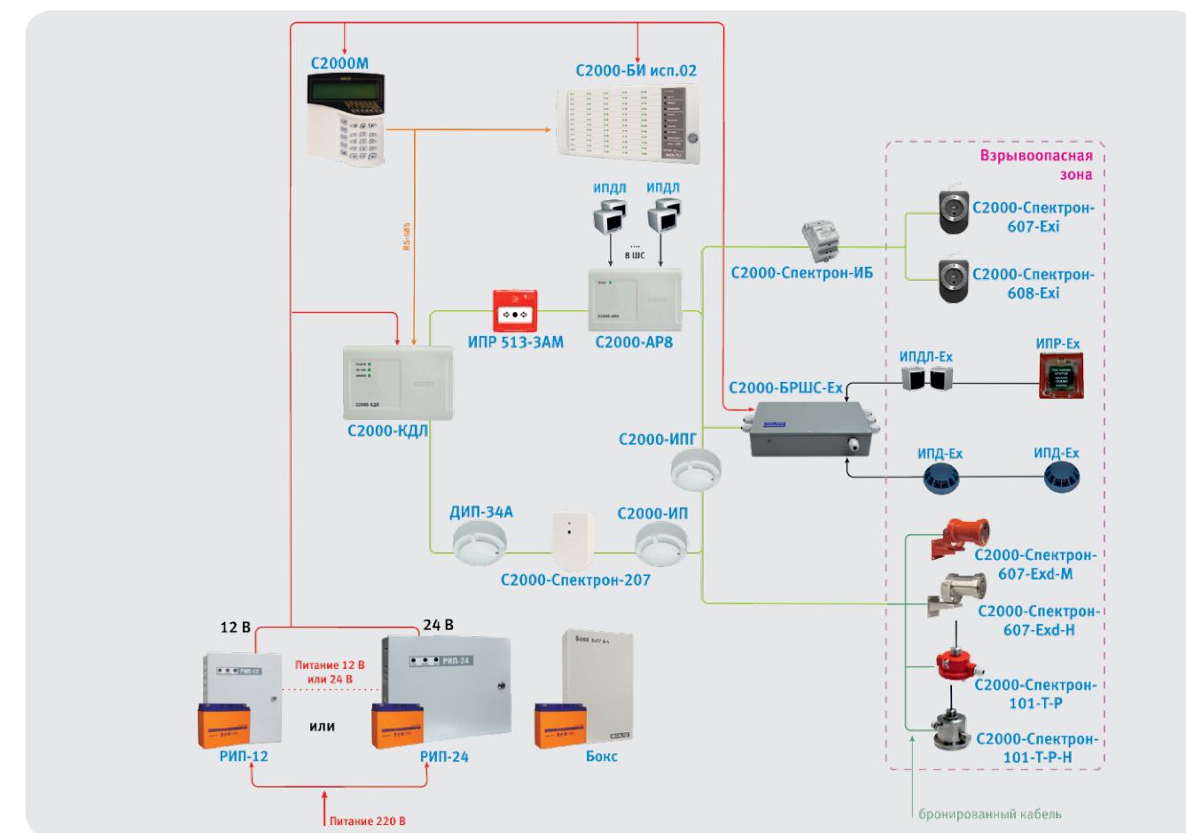
Рисунок 8. Взрывозащищённая система на базе адресно-аналоговой ПС
