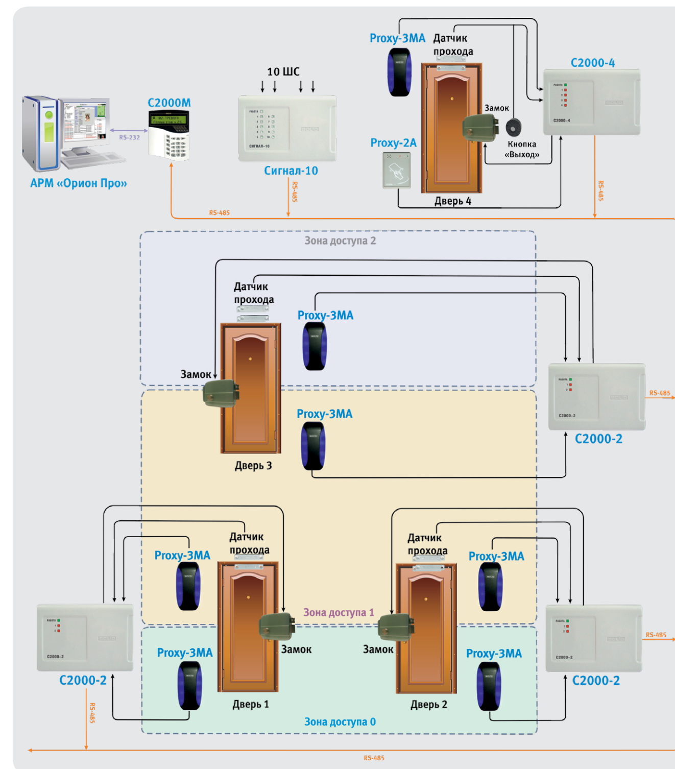
Рисунок 45. Сетевая СКУД с использованием программного обеспечения
