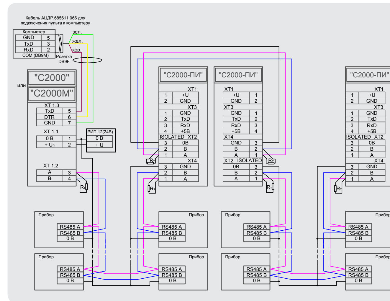
Рисунок 79. Увеличение длины линии RS-485 с помощью повторителей интерфейса
