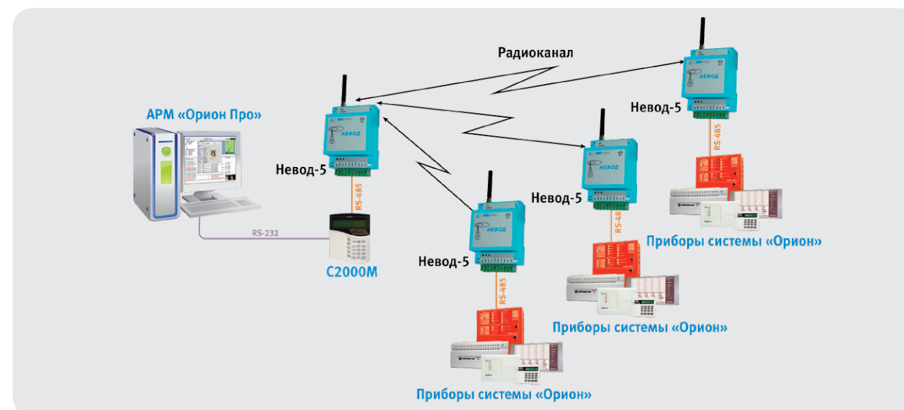
Рисунок 86. Структурная схема использования «Невод-5» с АРМ «Орион» и «C2000М», соединение «точка-многоточие»
