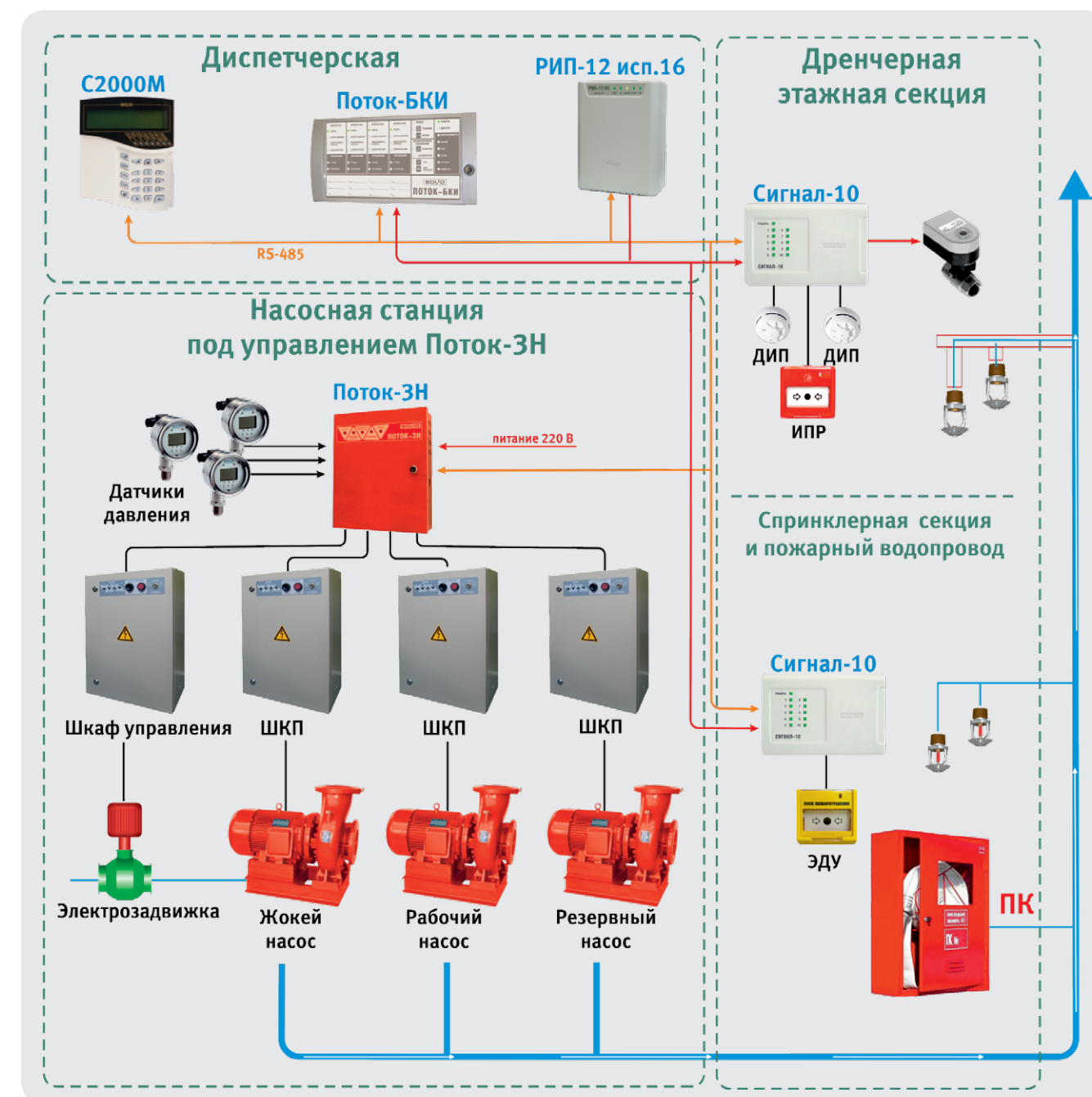
Рисунок 22. Система водяного пожаротушения с дренчерной секцией и пожарным водопроводом
