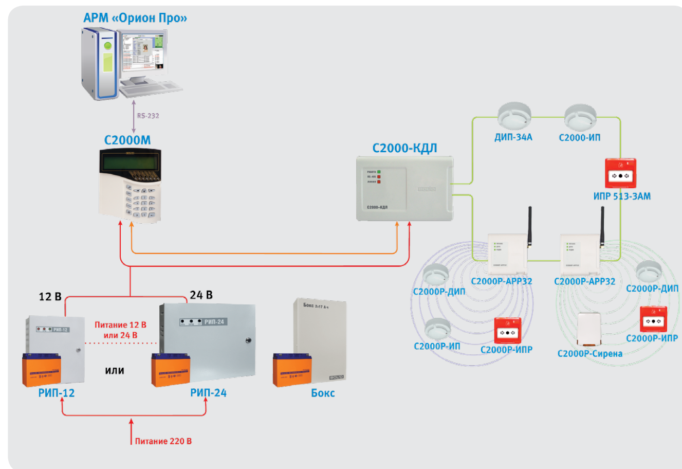
Рисунок 7. Радиоканальное расширение адресно-аналоговой системы пожарной сигнализации
