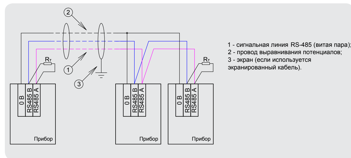
Рисунок 78. Схема подключения приборов к магистральному интерфейсу RS-485
