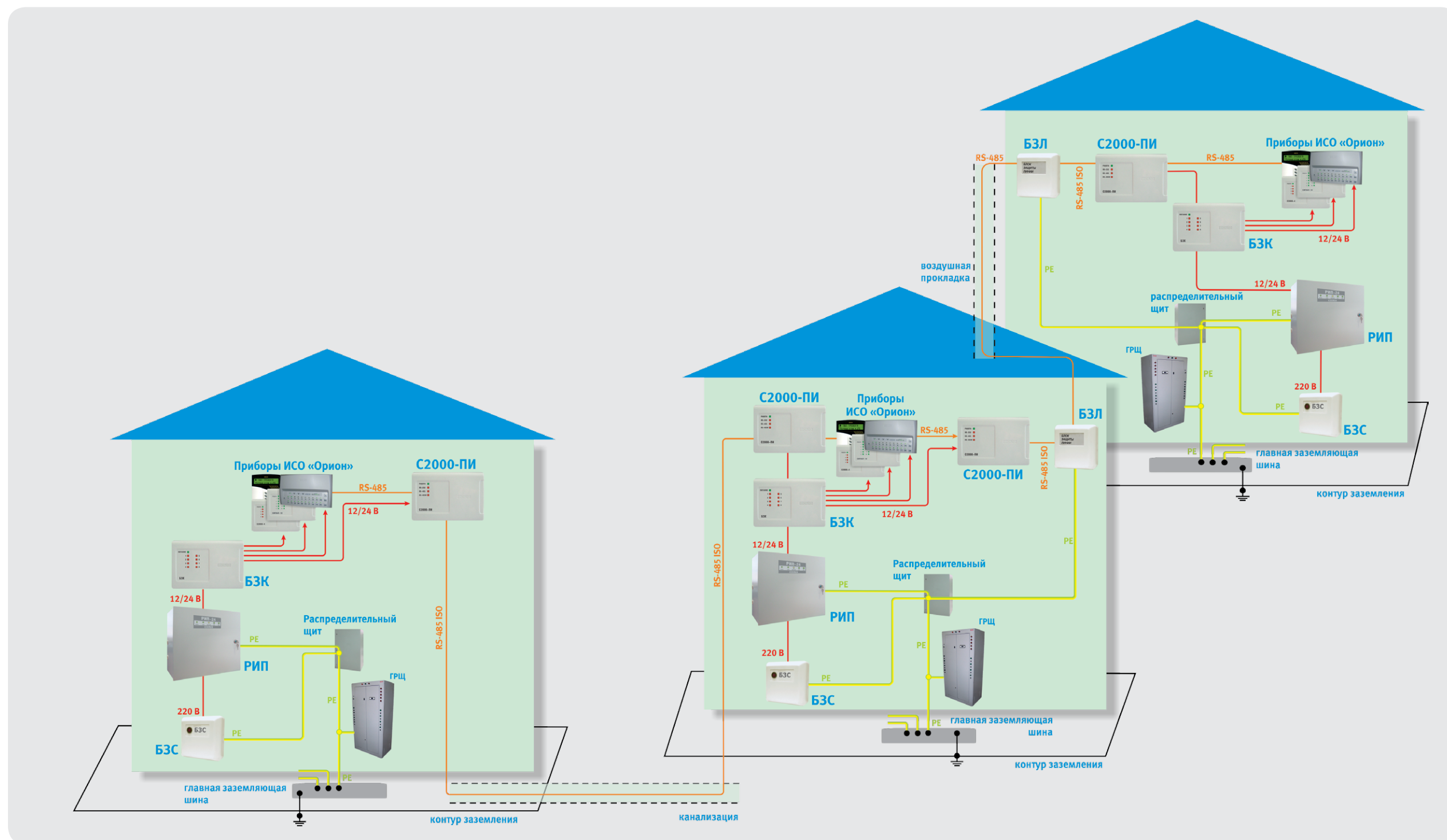
Рисунок 89. Схема подключения приборов с защитой интерфейса RS-485 от перенапряжений
