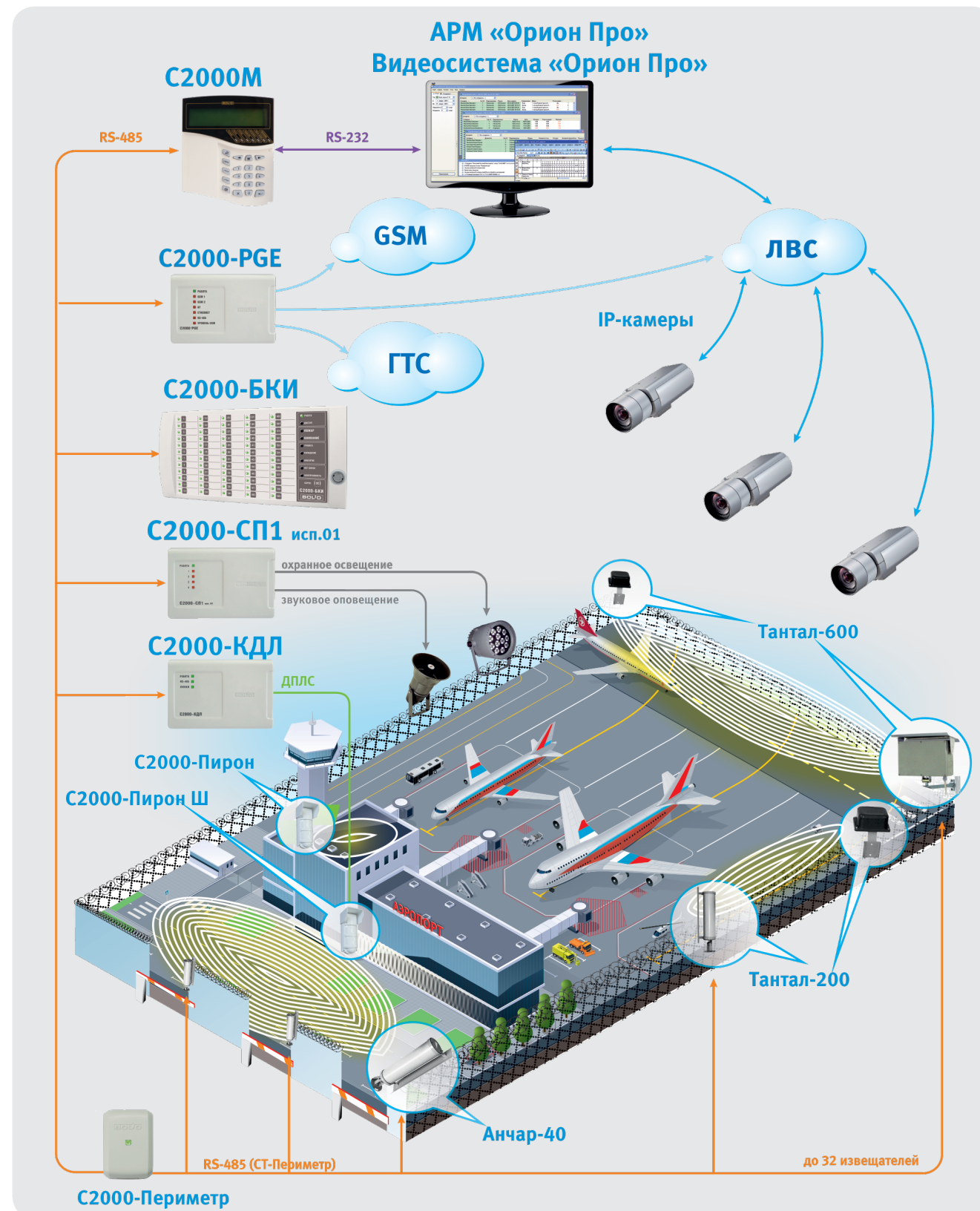
Рисунок 34. Система охраны периметра
