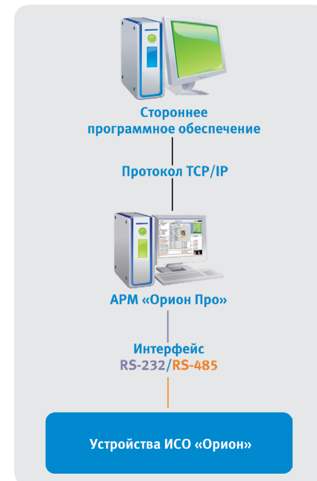
Рисунок 65. Интеграция с устройствами посредством интерфейса «Модуля управления» в АРМ «Орион Про»
