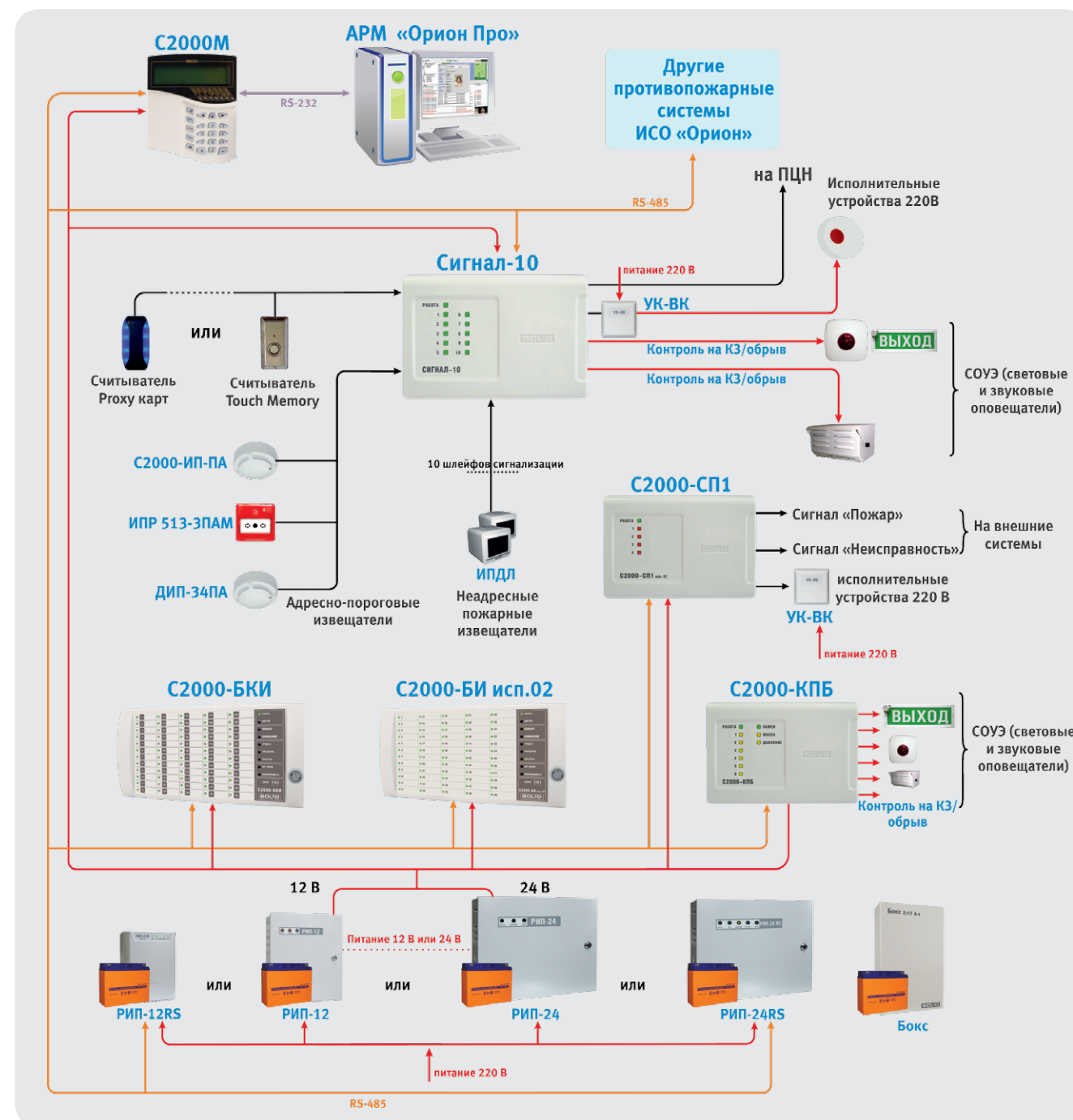
Рисунок 5. Адресно-пороговая система пожарной сигнализации с использованием блока «Сигнал-10»
