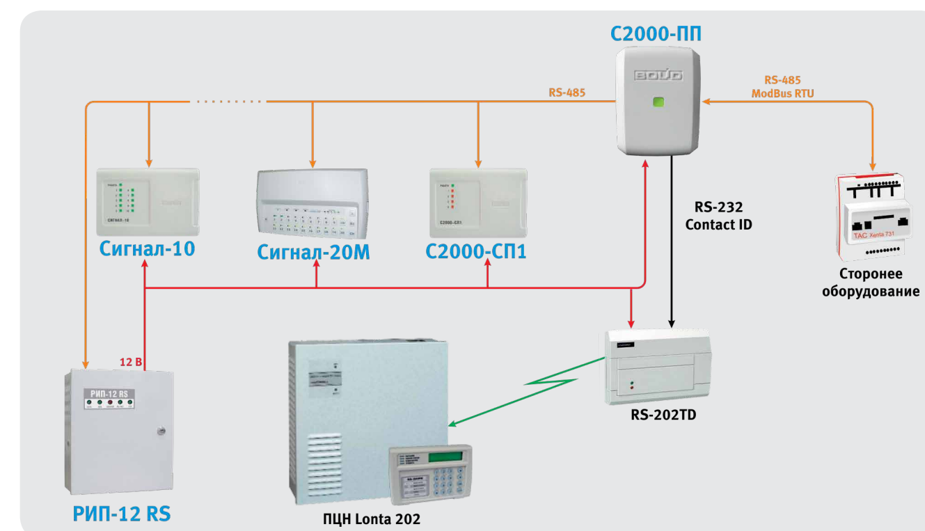
Рисунок 62. Применение «С2000-ПП» в ведущем режиме
