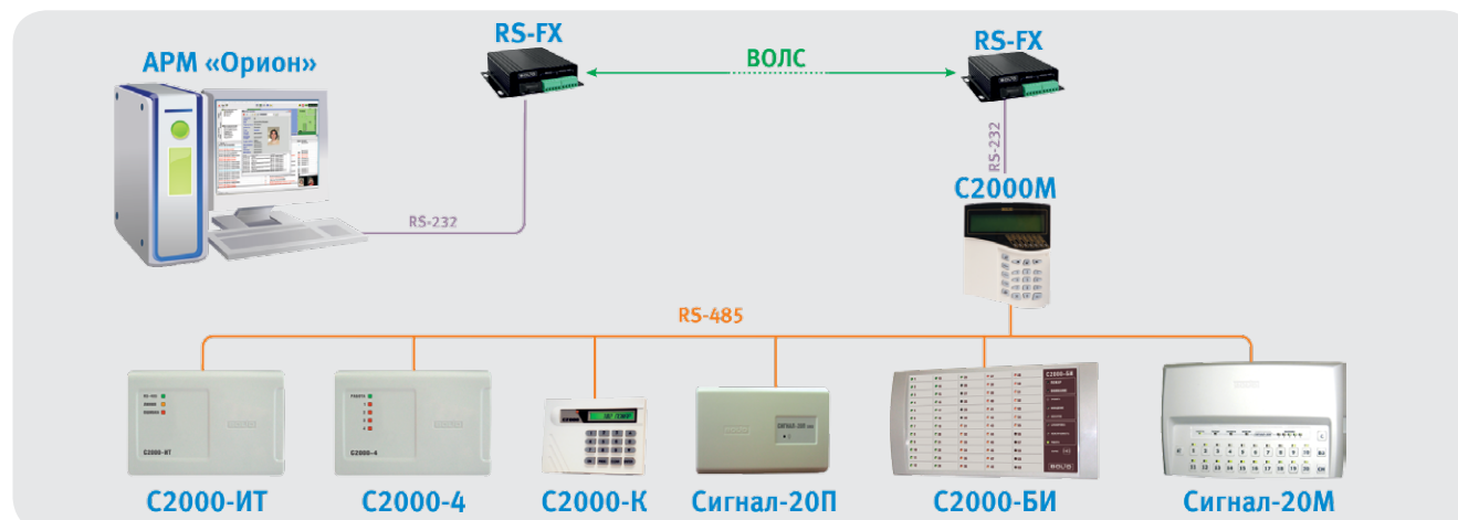
Рисунок 74. Типовая схема работы преобразователей RS-FX по протоколу «Орион Про»
