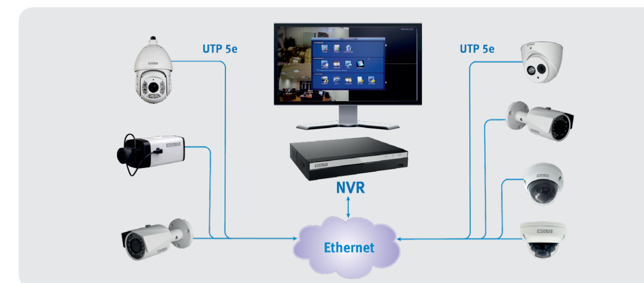
Рисунок 49. Сетевое видеонаблюдение с локальным рабочим местом
