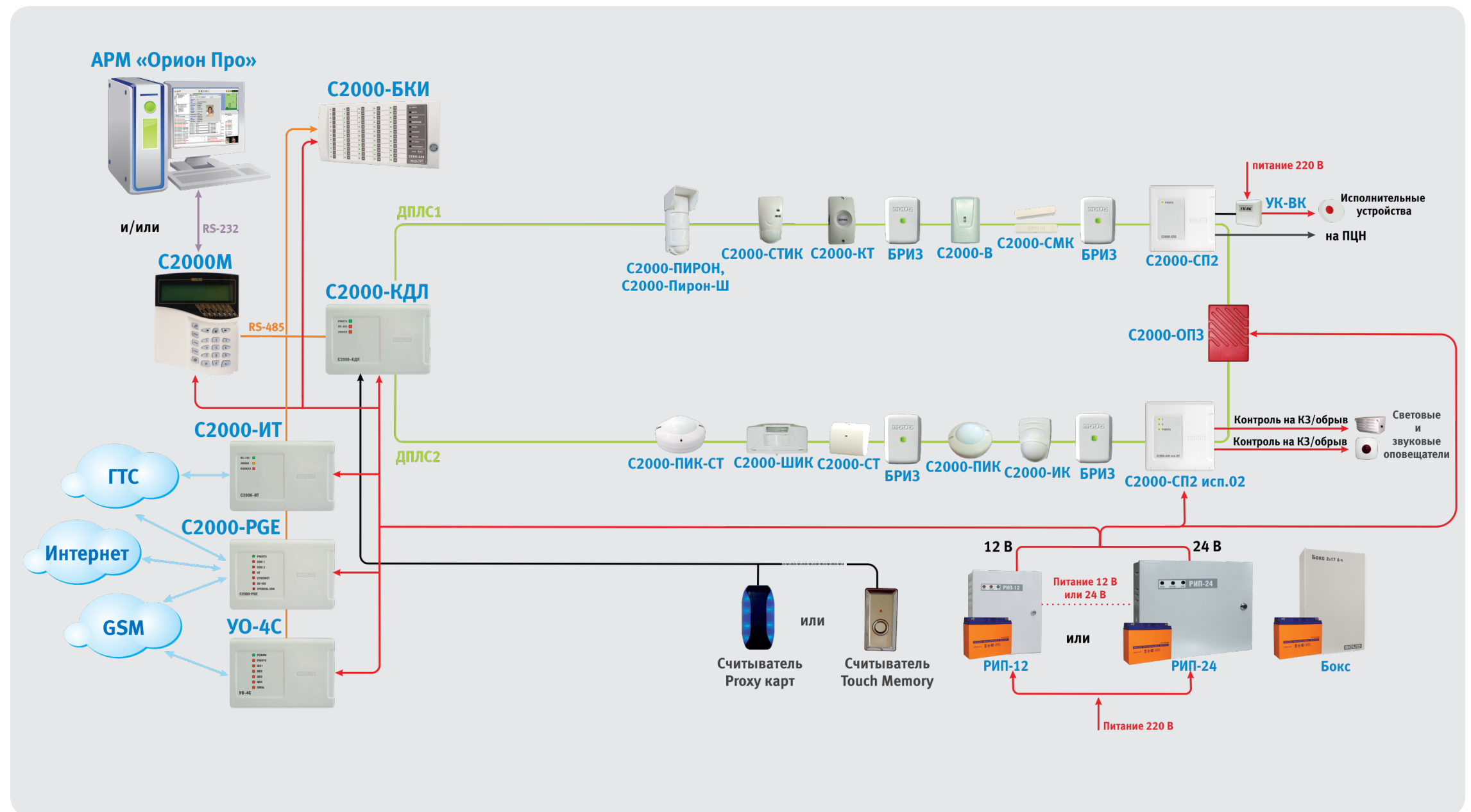
Рисунок 31. Адресная система охранной сигнализации
