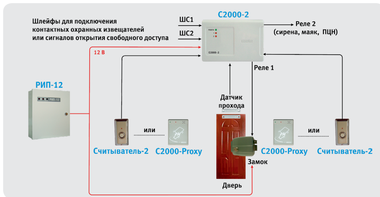
Рисунок 37. Режим работы «Одна дверь на вход/выход»
