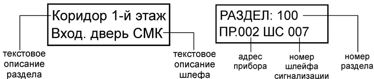
Рисунок 3.6. Примеры экрана пульта при нажатии клавиши «2»
