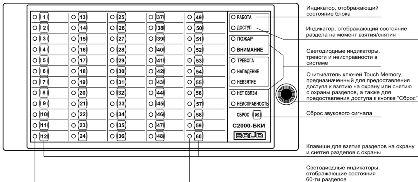
Рисунок 3.10. Внешний вид, органы индикации и управления блока «C2000-БКИ»
