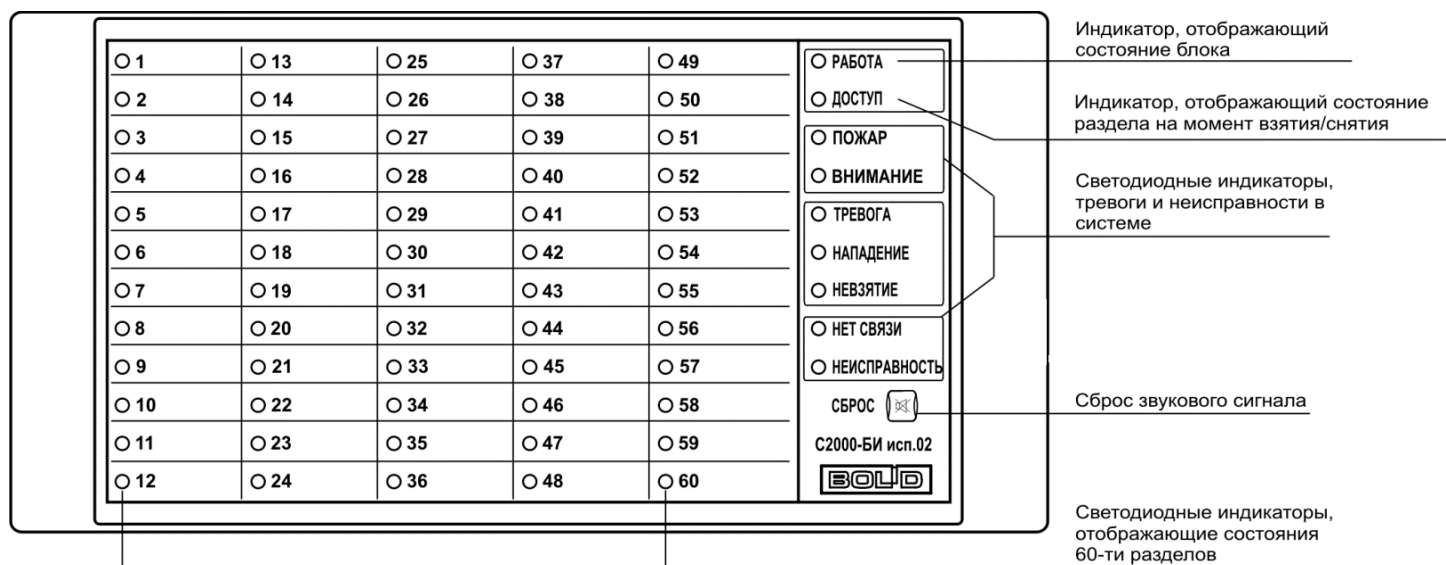
Рисунок 3.9. Внешний вид, органы индикации и управления блока C2000-БИ исп.02
